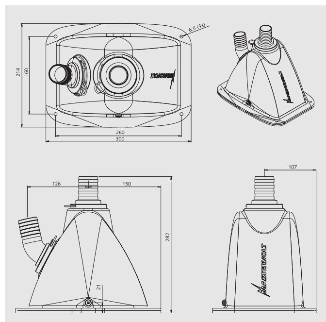
Abmessungen in mm des Delta Schalldämpfers/Wassersammlers.
