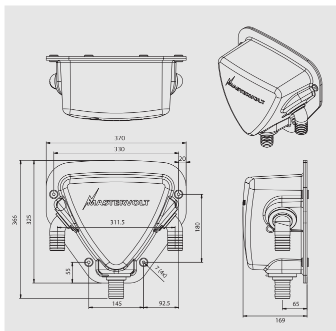
Abmessungen in mm des Delta Abgas-/Wasserabscheiders.
